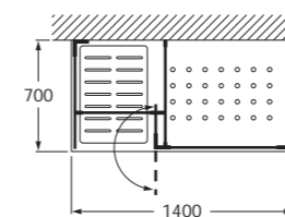
7M313R4712 Sprchový kout k vaničke Malta Walk-In rohový, pravý, 140 x 200 cm, barva výplně transparent, barva hliníkového profilu stříbrná
